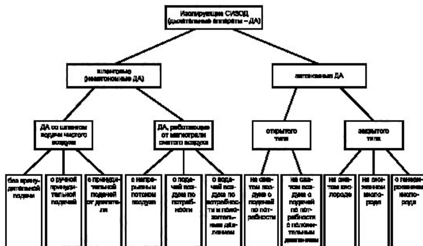
Рисунок 4 — Классификация изолирующих средств индивидуальной защиты органов дыхания
