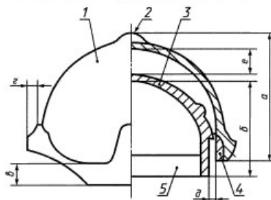
Схематическое изображение конструкции каски
